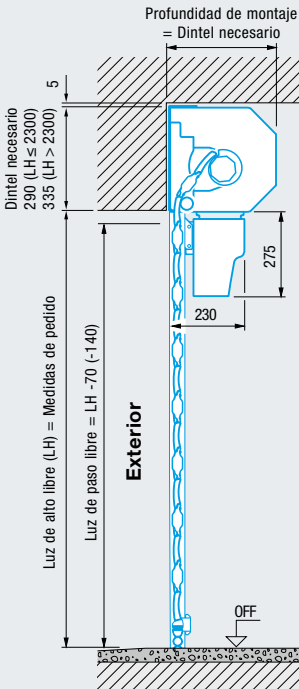
Montaje detrás del hueco
