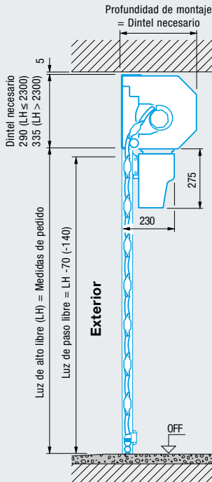
Montaje en el hueco
