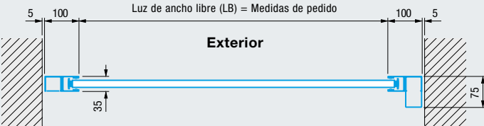
Montaje en el hueco
